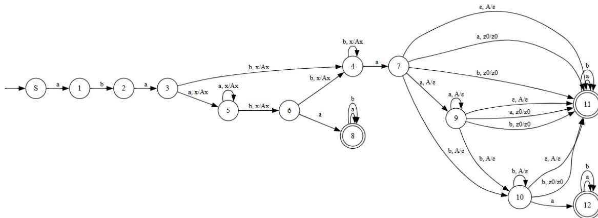
Рис. 3: ветвь DPDA по пути aba
