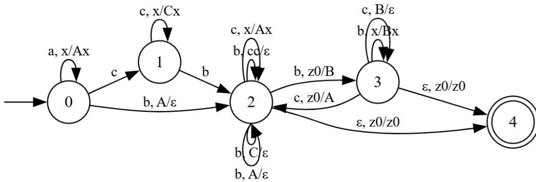
Рис. 1: PDA-автомат
